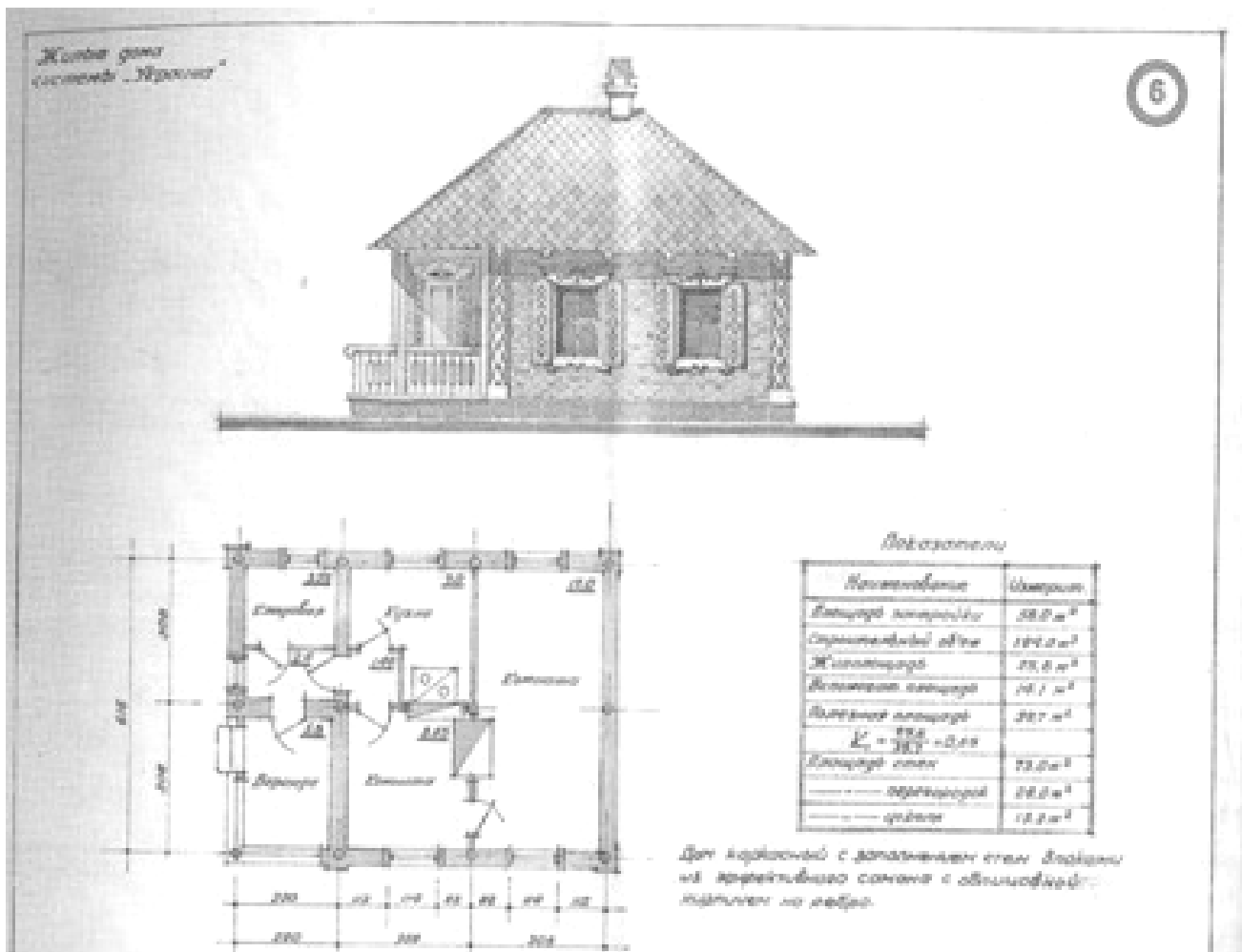
Рис. 1. Проект стандартного збірного будинку системи «Україна»
