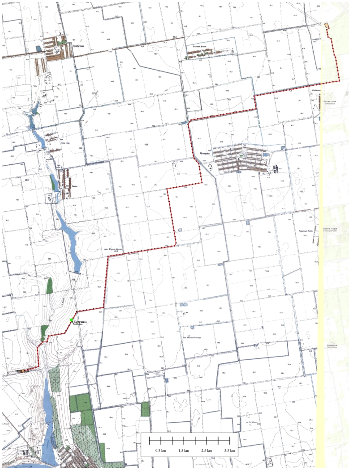
Рис. 1. Маршрут-схема ЛЕП та досліджуваної території.
