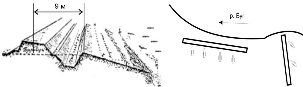
Рис 1. План батареї
